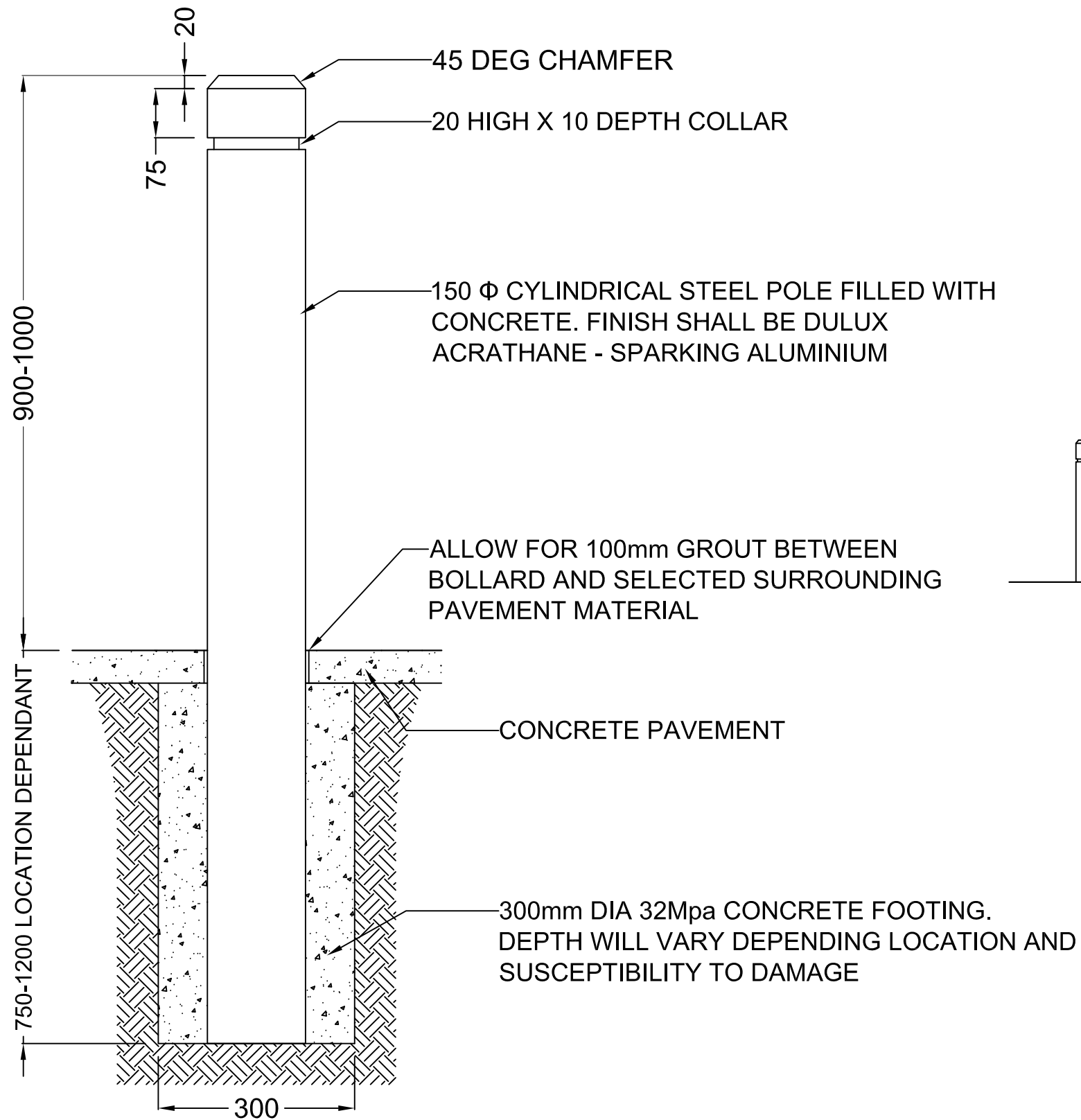
ELEVATION
